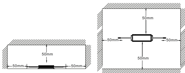
Sposób montażu oraz przestrzeń wokół zasilacza
